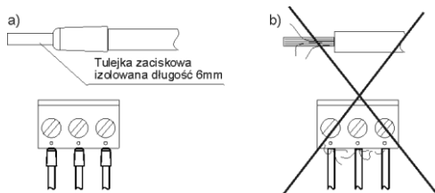
Rys. 5 Zabezpieczanie końców przewodów: a) prawidłowe, b) nieprawidłowe
