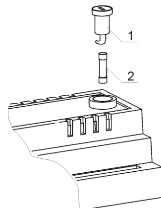
Rys. 6 Wymiana bezpiecznika; gdzie: 1 – bezpiecznik, 2 – oprawka bezpiecznika
